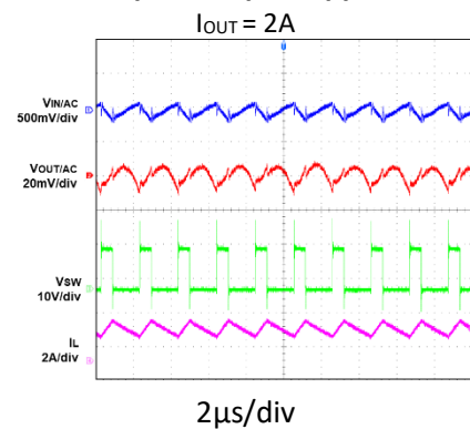
Input/Output Ripple
